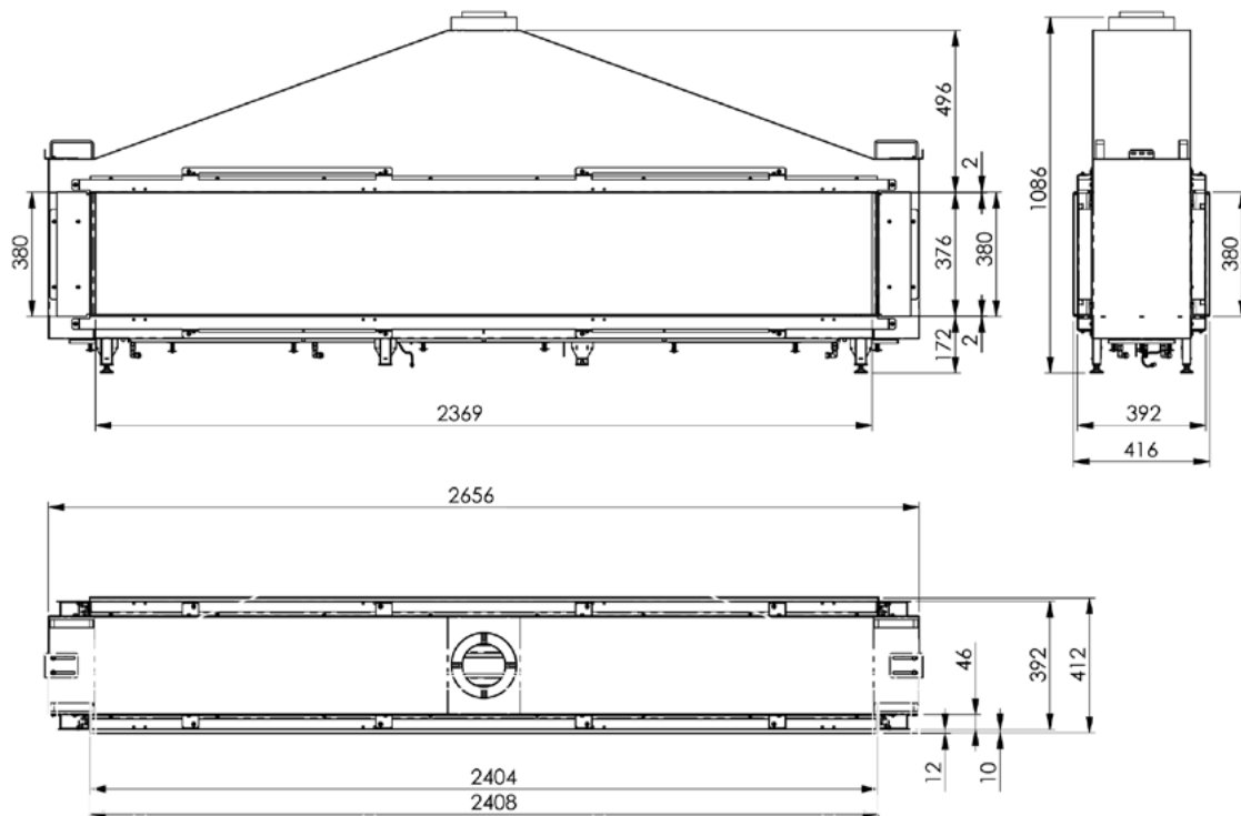
VISIONE DEL FUOCO (L X H): 237 X 38 CM
