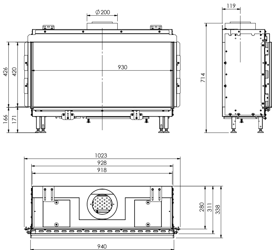
VISIONE DEL FUOCO (L X H): 93 X 42 CM
