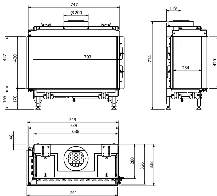
VISIONE DEL FUOCO (L X H X P): 70 X 42 X 23 CM
